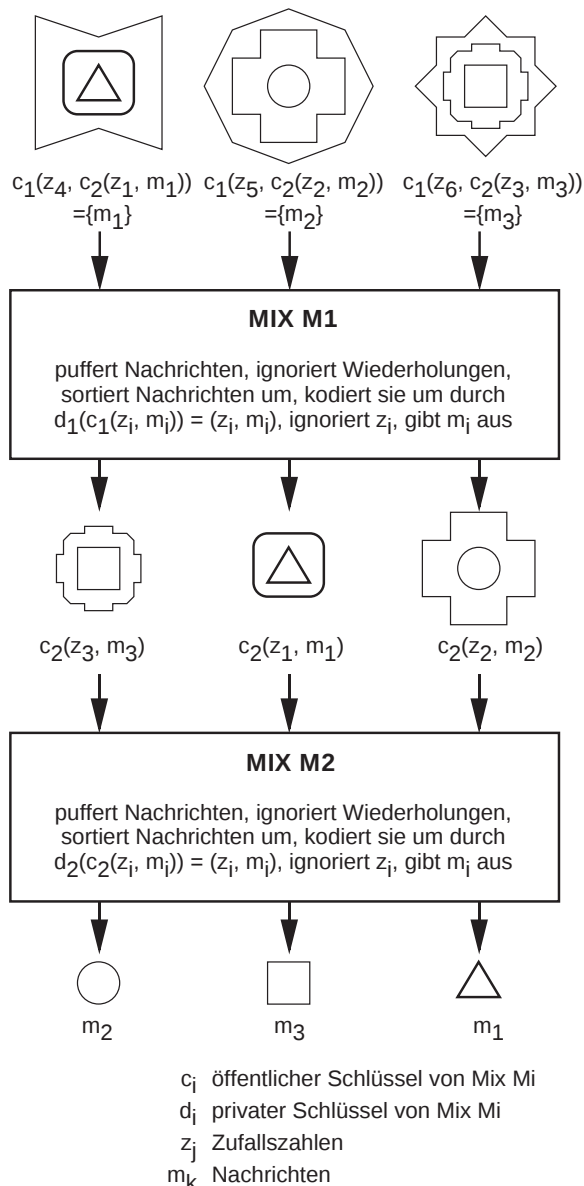
Bild 2. Umkodieren gemixter Nachrichten
