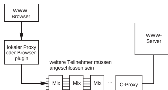
Bild 4. Architektur des Dienstes
