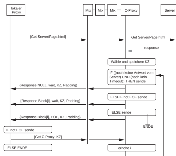
Bild 5. Protokoll zwischen lokalem und C-Proxy
